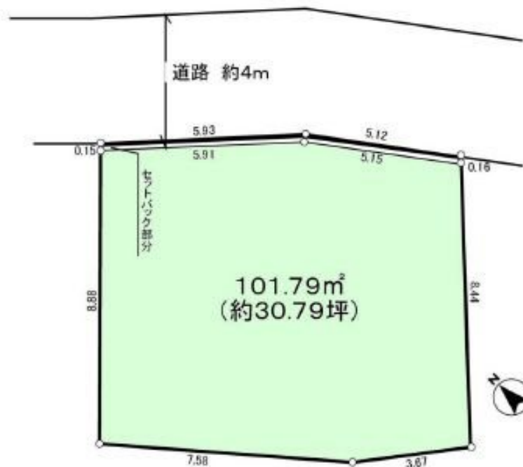
【区画图】
