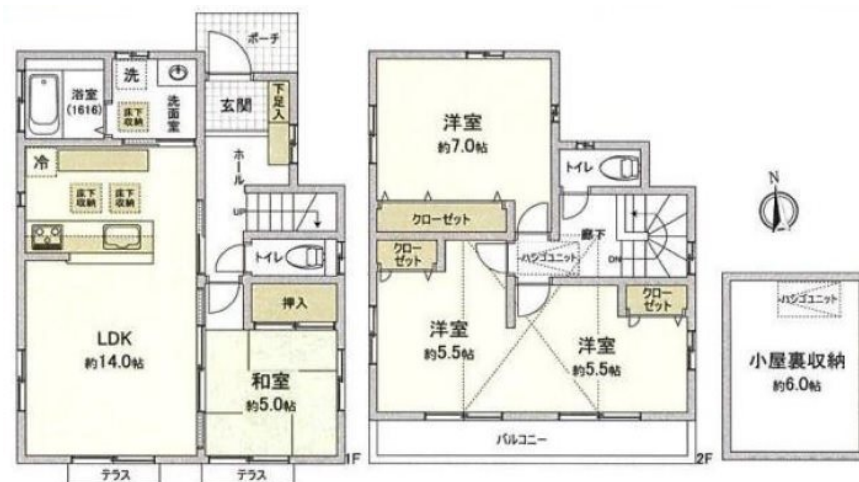
【間取り図】
